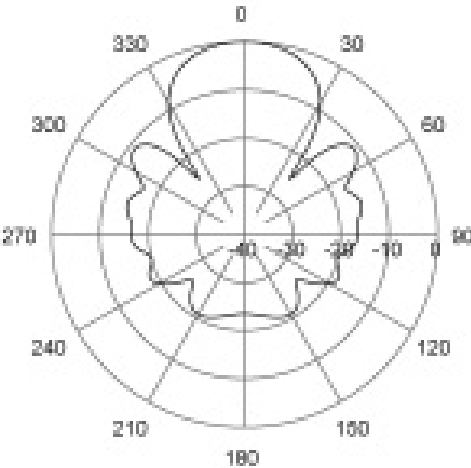
H-Plane | 415 MHz
