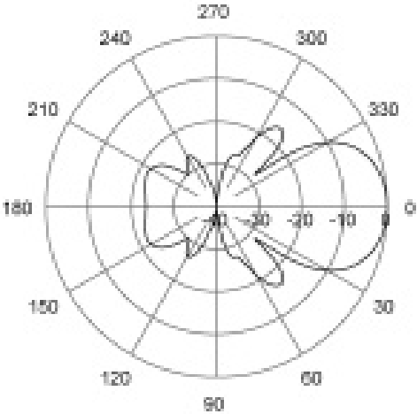
E-Plane | 415 MHz
