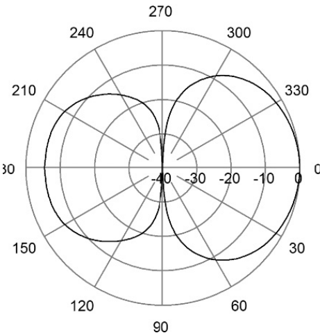
E-Plane | 225 MHz
