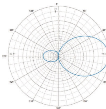
E-Plane | 165 MHz
